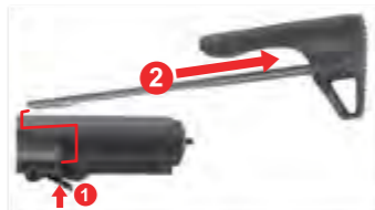
1. 按下伸縮托鈕 2. 移除槍托
