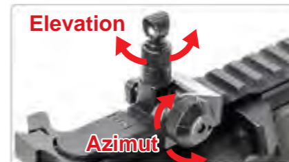
Azimuth (réglage gauche/droite) Elevation (réglage haut/bas)
